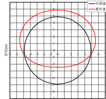
図-3 トンネル変位分布 (テール脱出 12R 後)
