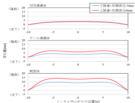
図-6 地表面鉛直変位 (上限値+初期変位 0mm, 下限値+初期変位-5mm)
