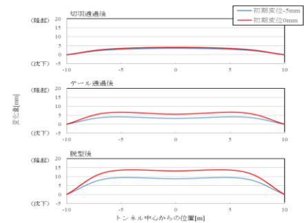
図-5 地表面鉛直変位
