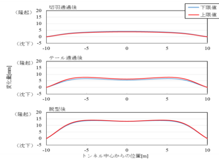
図-4 地表面鉛直変位 (上限値, 下限値)
