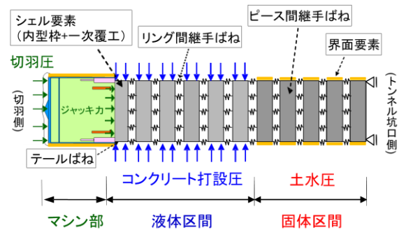
図-1 解析モデルの概要図
