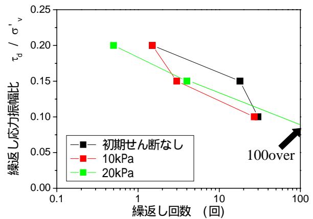
Fig.11 液状化強度曲線
