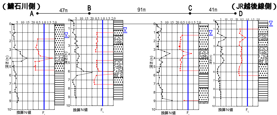
Fig. 4 液状化判定
