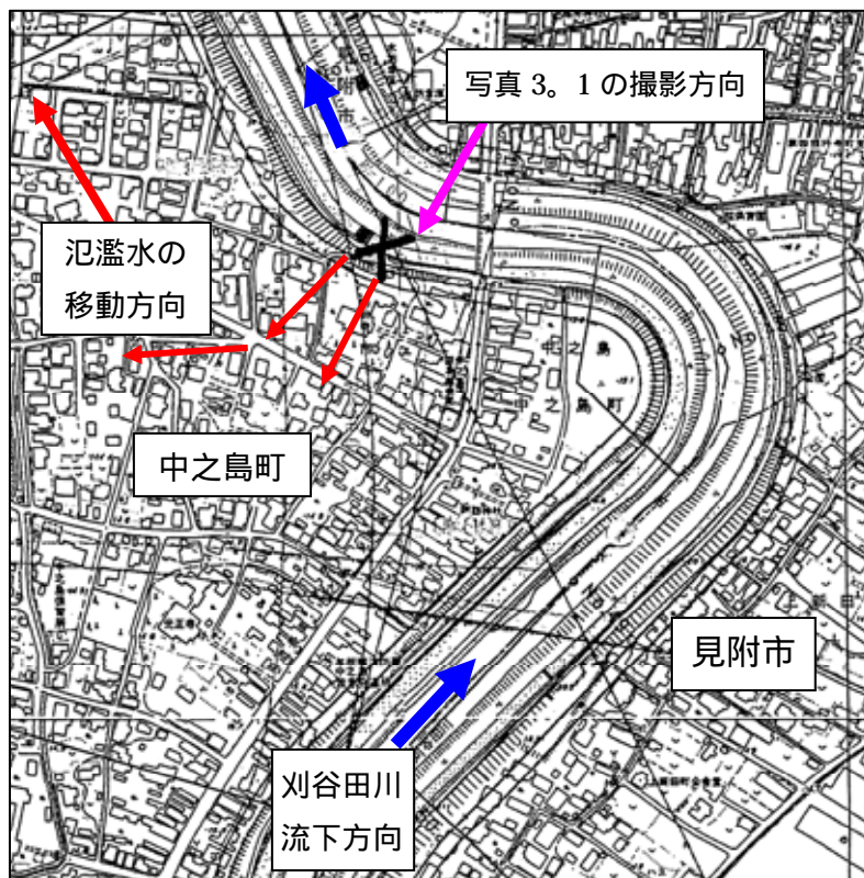
図 4-2 中之島町破堤点近くの刈谷田川（×点：破堤点）
