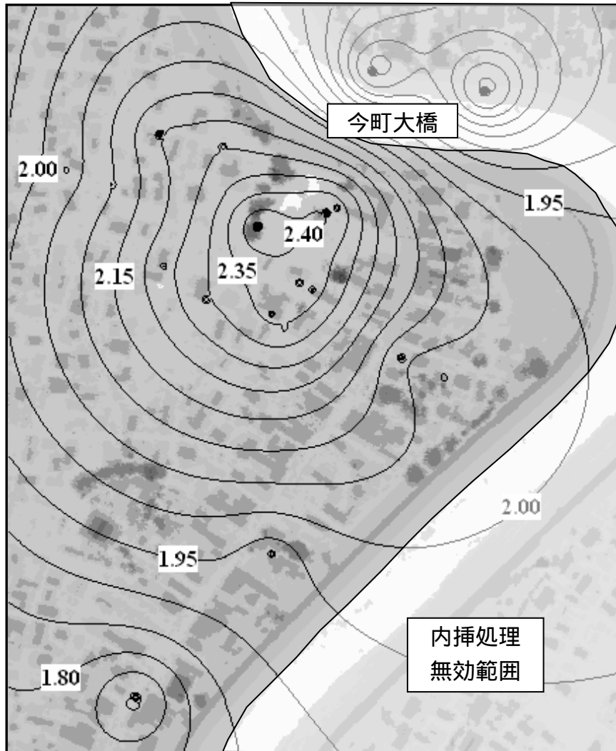
図 4-5 秋田大学松富らの現地測量に基づく内挿された 痕跡水位分布 (m) 縦 : 594m、横 515m
