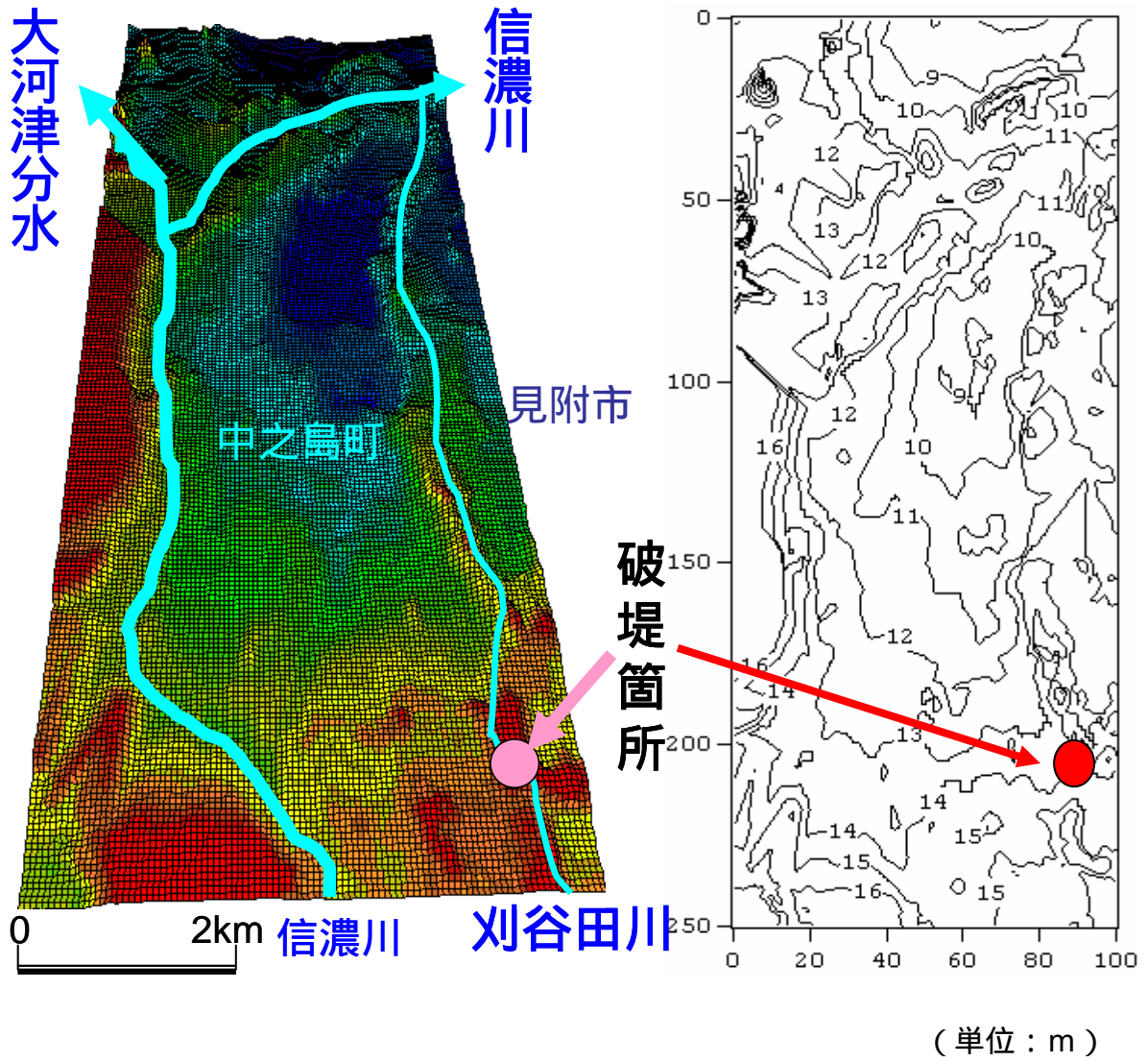
図 4-7 計算領域 (左：鳥瞰図、右：等高線図)
