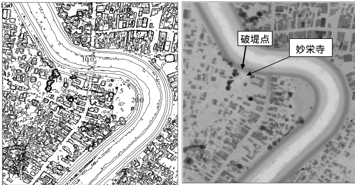
図 4-3 災害直後に航空写真測量より計測された中之島町破堤点近傍の DEM （今町大橋は除去されている） 縦:1101m、横:1001m
